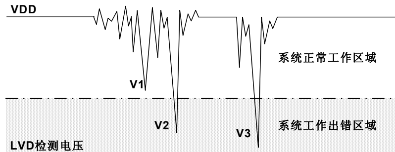
掉电复位示意图
